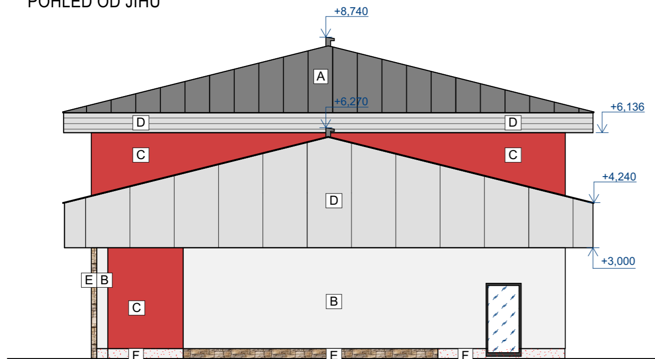
POHLED OD JIHU
